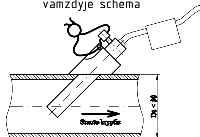
Temperatūros jutiklio montavimo vamzdyje schema
